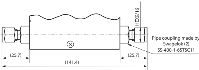
1/4" Swagelok connection type (option)
