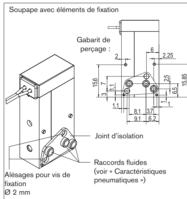
Figure : plan de montage
